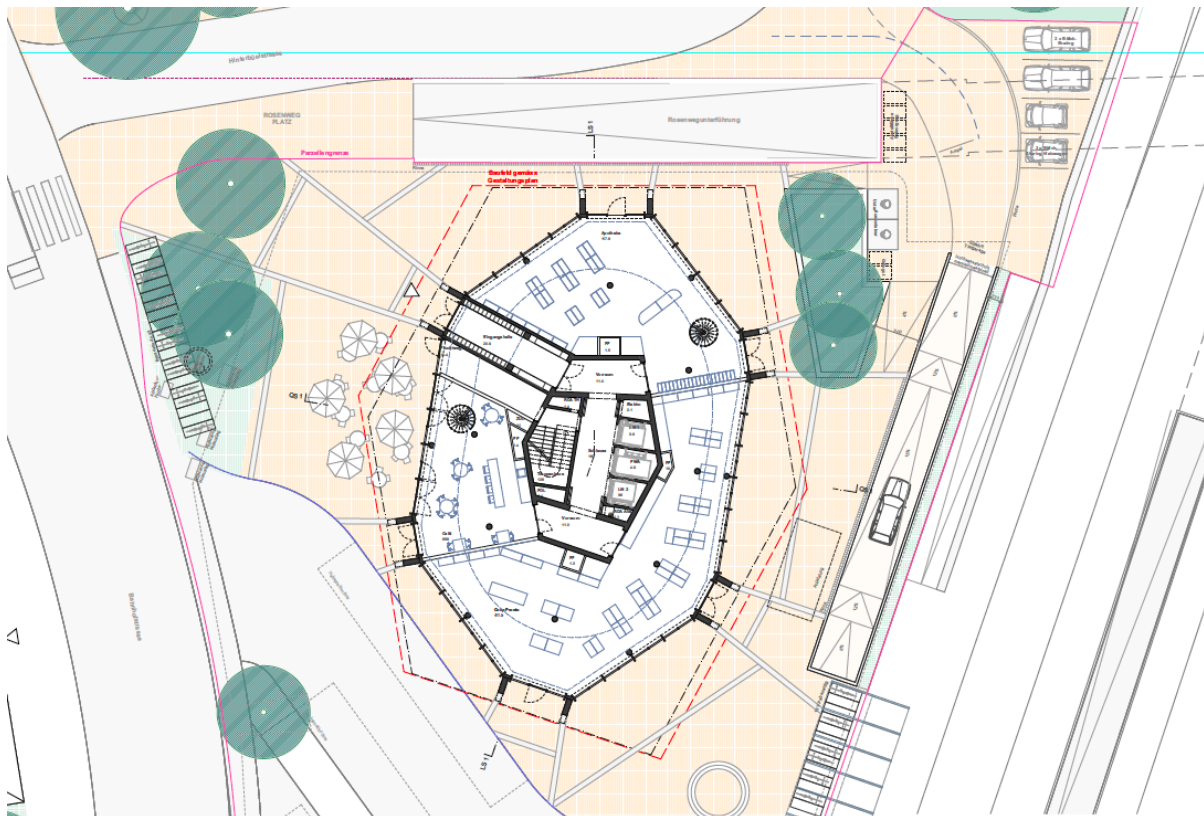
Abbildung 1: Übersichtsplan EG (pool Architekten, 2022)
