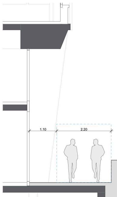
Lichtraumprofil in Übereinstimmung mit den Anforderungen gemäss SN 40 201
